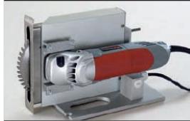
Отрезной агрегат для продольной резки
