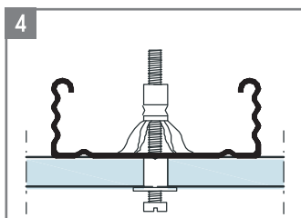
Дюбель для пустотелых конструкций
