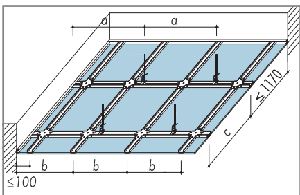
Металлический каркас подвесного потолка П 113
