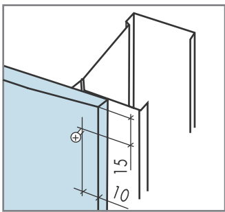
Правильное крепление листов
