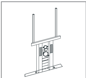
Металлическая рама для навеса сантехнического оборудования
