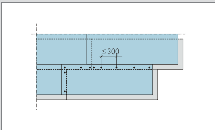
Схема крепления элементов пола из КНАУФ-листов
