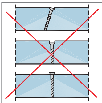
Неправильная установка шурупа
