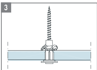
Дюбель мультифункциональный
