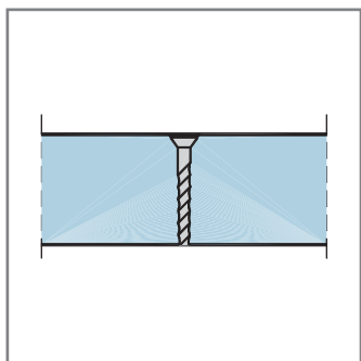
Правильная установка шурупа
