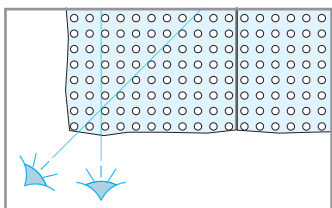
3. Плиты монтируются так, чтобы ряды перфорации по диагонали, в продольном и поперечном направлениях не имели смещений
