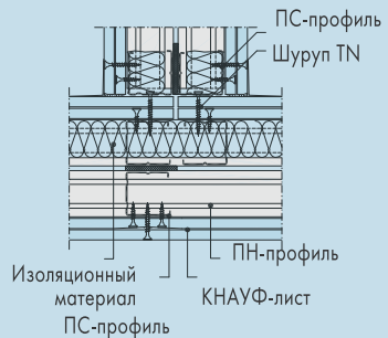
Формирование T-образного соединения перегородки
