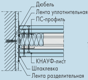
Сопряжение перегородки с капитальной стеной
